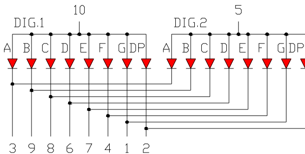
OPS-D3920LE-2-STT(R)-1.0-G(B)W (Common Anode)
